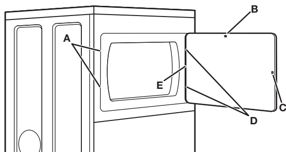
A. Fiches B. Pilon de retenue de la porte (porte pleine) C. Pilon de retenue de la porte (porte avec hublot) D. Charnières E. Étiquette de gâche de porte
