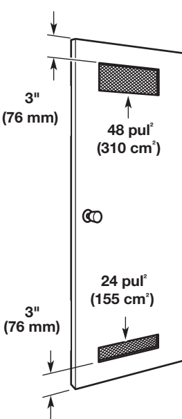
Tamaños mínimos aceptables de los ductos de la puerta del clóset
