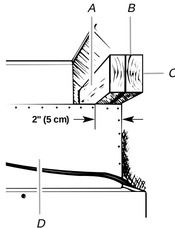
A. Deux panneaux de 2 po x 4 po x 32 po (5 cm x 10 cm x 81 cm) B. aux montants avec six vis no 8 x 3 po (7,6 cm). C. Couvercle du compresseur D. Distance entre le bas du panneau antibascullement et le plancher
