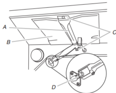
A. Brûleur du gril B. Répartiteur de flammes C. Vis D. Injecteur
