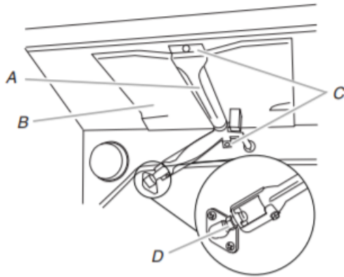
A. Brûleur de grill B. Répartiteur de flammes C. Vis D. Injecteur
