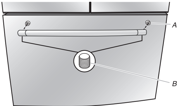
A. Tornillo de tope B. Tornillos de fijación dentro de la manija
