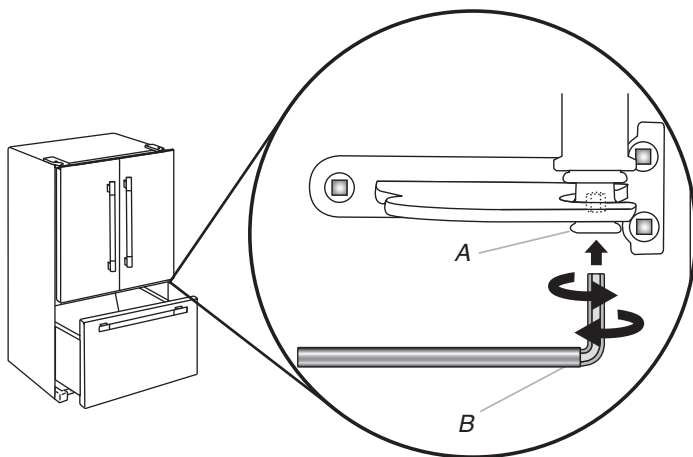
A. Pasador de bisagra inferior B. Llave hexagonal de 1/8" (3,2 mm)
