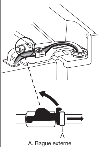
Raccord de tuyau du distributeur d'eau
