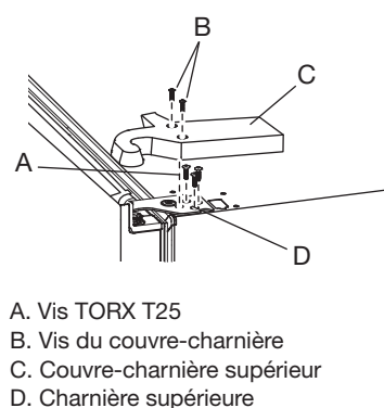
Charnière supérieure droite
