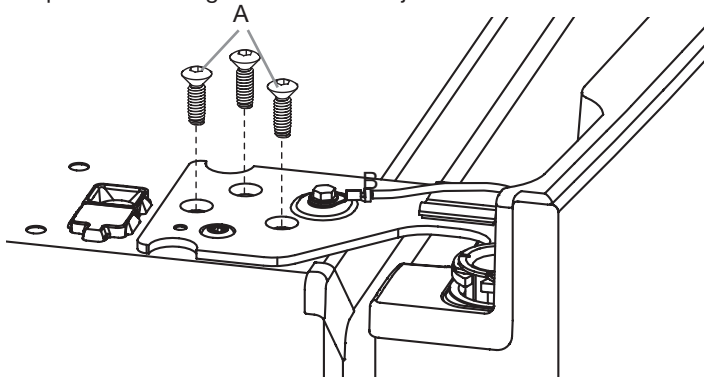
A. Tornillos TORX T25 B. Cable a tierra (no lo quite)
