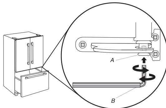
A. Axe de charnière inférieure B. Clé à tête hexagonale de 1/8" (3,2 mm)
