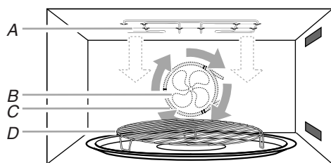
A. Élément de cuisson au grill C. Élément de convection B. Ventilateur de convection D. Grille de convection
