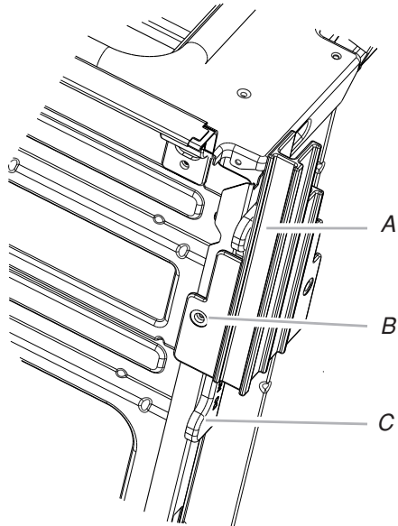
A. Front foot B. #8-18 x ¾" screw C. Spacer
