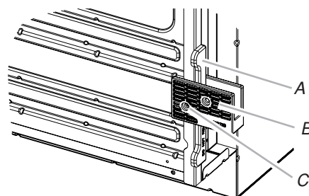
A. Spacer B. Foot C. #8-18 x ¾" screw
