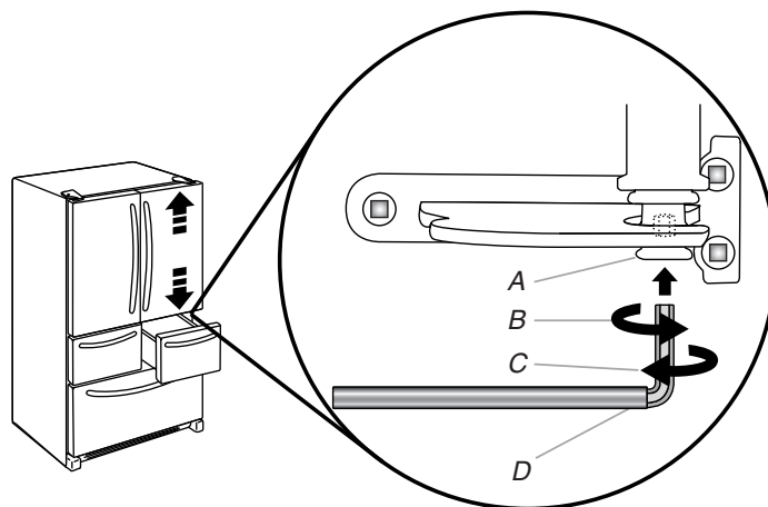
A. Bottom hinge pin
