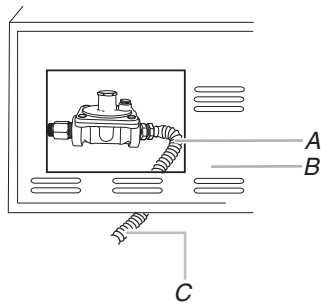
A. Conduit de raccordement flexible neuf, pour l'utilisation à l'extérieur (homologation CSA International) B. Arrière du gril C. Vers canalisation locale de gaz propane
