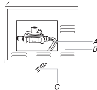
A. Conduit de raccordement flexible neuf, pour l'utilisation à l'extérieur (homologation CSA International) B. Arrière du gril C. Vers canalisation locale de gaz naturel
